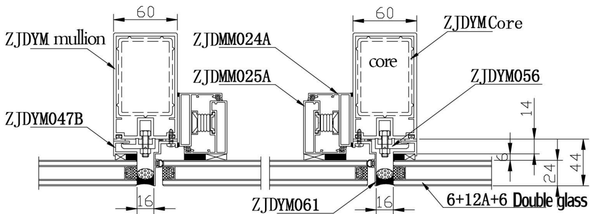
A-A
