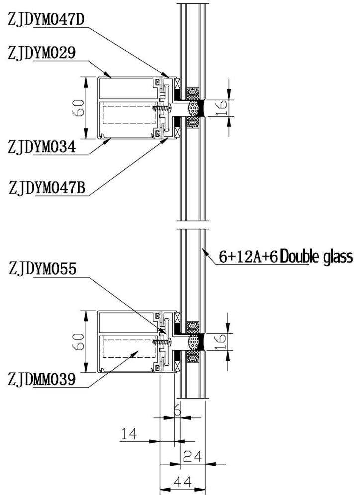
B-B
