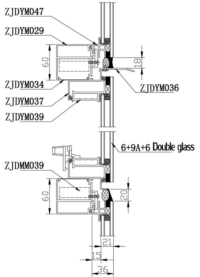
B-B
